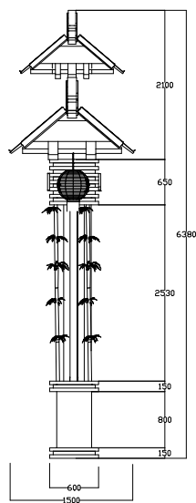
POTONGAN DESAIN GAPURA SKALA 1 : 100
