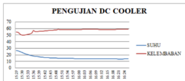
Gambar 7 Grafik pengujian Dc cooler.
