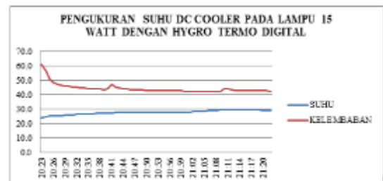
Gambar 17 Pengukuran suhu dc cooler pada lampu 15 watt.
