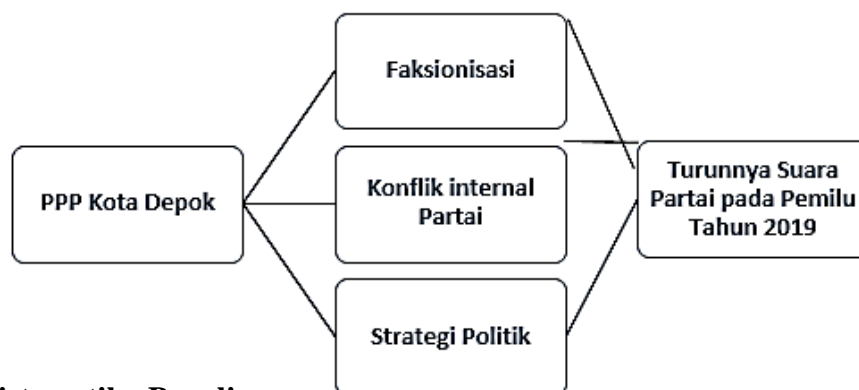
Gambar 3.1 Kerangka Berpikir
