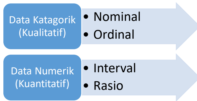
Gambar. Tipe Data Statistik
